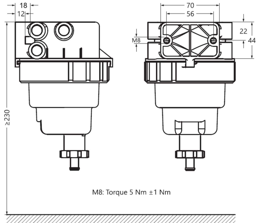
Abbildung 7: Montagemaße
