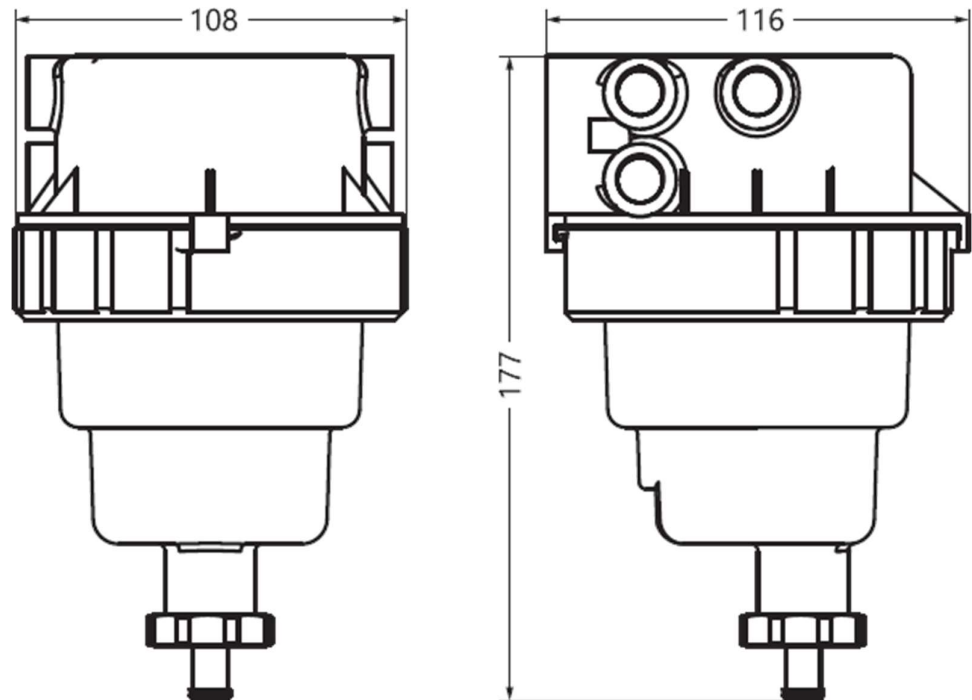
Abbildung 2: Abmessungen
