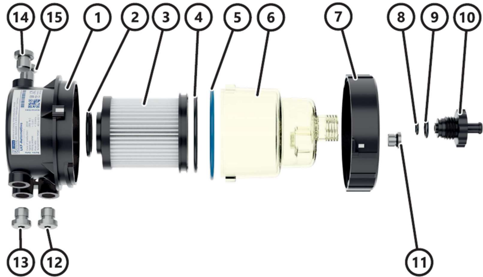
Abbildung 4: Einzelteile des Filters
