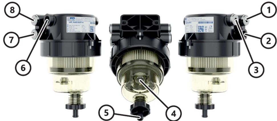
Abbildung 9: Mechanische Anschlüsse
