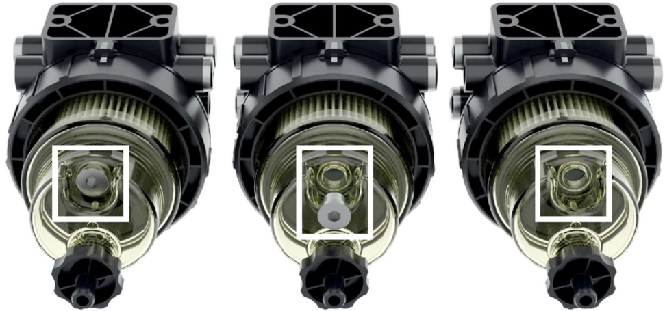
Abbildung 14: Einschraubgewinde für den Wassersensor
