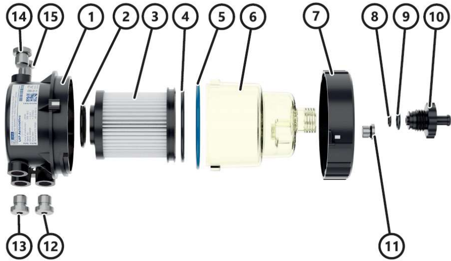
Abbildung 18: Einzelteile des Filters
