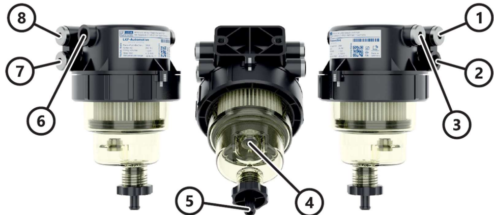
Abbildung 6: Mechanische Anschlüsse
