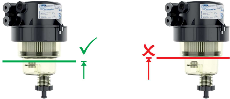
Abbildung 19: Zulässiger Maximalwasserstand
